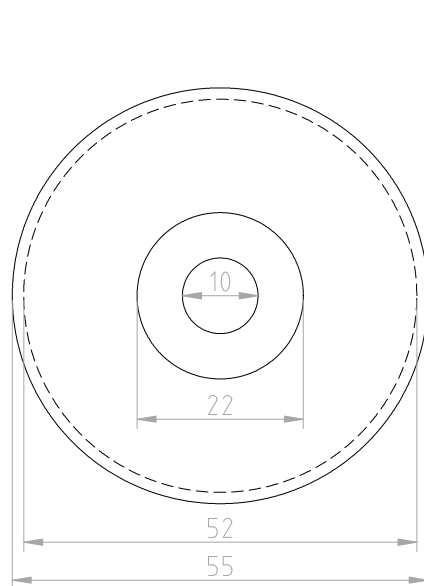
Ruedas
