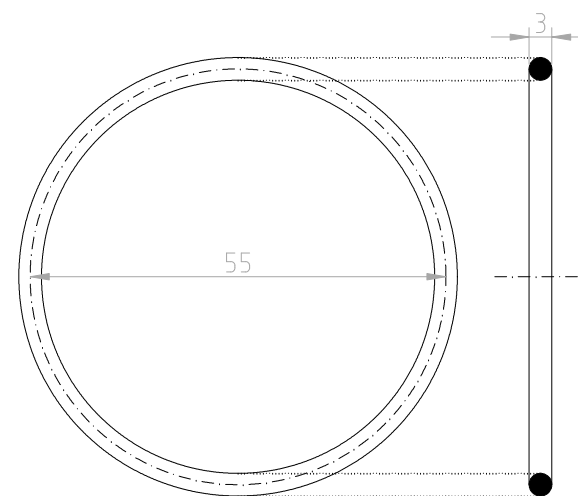
Frontal
