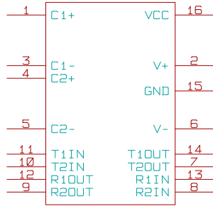
MAX232
